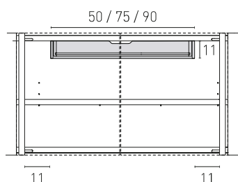
Modulo cassetto sottopiano
