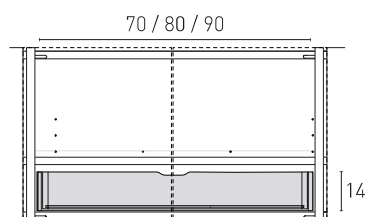
Modulo cassetto interno
