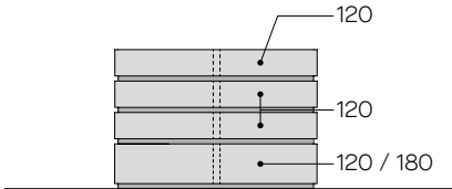
Stack max 4 x 1200 aligned elements or 3 x 1200 and 1 x 440 / 600 / 720 / 900 elements Apilar máx. 4 elementos 1200 alineados o 3 de 1200 y 1 de 440 / 600 / 720 / 900
