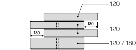
Stack max 4 x 1200 elements offset by max 180 or 3 x 1200 and 1 x 440 / 600 / 720 / 900 elements Apilar máx. 4 elementos 1200 escalonados máx. 180 o 3 de 1200 y 1 de 440 / 600 / 720 / 900
