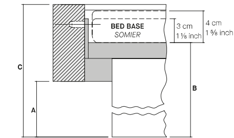
Crossbar for 3/4 cm bed base Travesaño para somier de 3/4 cm
