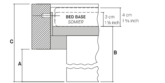
Crossbar for 3/4 cm bed base Travesaño para somier de 3/4 cm
