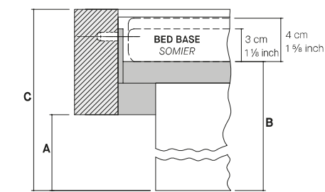
Crossbar for 3/4 cm bed base Travesaño para somier de 3/4 cm
