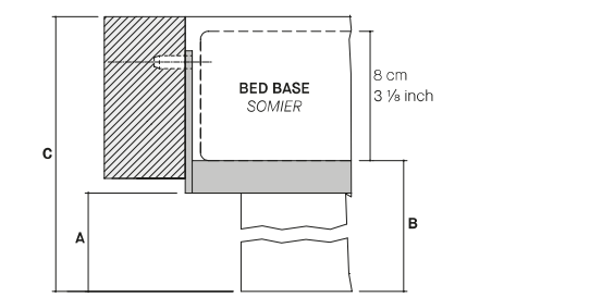
Crossbar for bed base up to 8 cm Travesaño para somier hasta 8 cm
