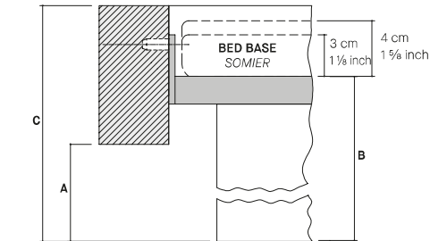
Crossbar for 3/4 cm bed base Travesaño para somier de 3/4 cm
