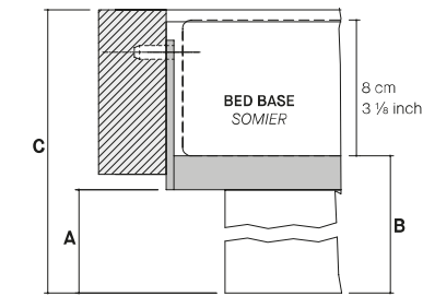
Crossbar for bed base up to 8 cm Travesaño para somier hasta 8 cm
