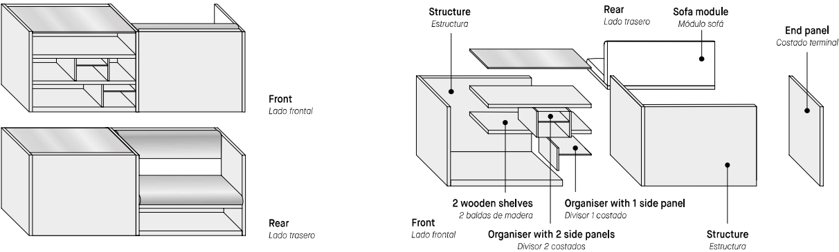
Example of adjacent/inverted structure Ejemplo estructura adosada/invertida
