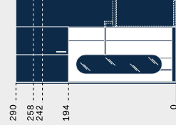
Nicchia con specchio Recess with mirror
